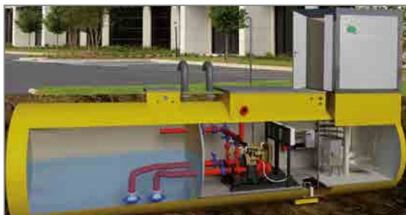
Sistema antincendio da interno completo di riserva idrica e vano tecnico secondo norme vigenti
