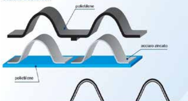
Sezione trasversale
